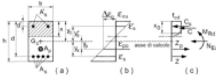
Fig. 4.1.4 - Sezione pressoinflessa
