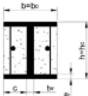
Fig. 7.6.1 - Rapporti dimensionali
